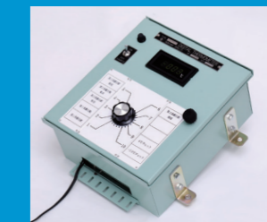
■ デジタル温度計(切換スイッチタイプ) DMH / DMR型 DM表示器と切換スイッチタイプの温度計です。盤埋込式 / 壁掛式があります。入力はK熱電対、Pt100他電圧電流にも対応しています。
